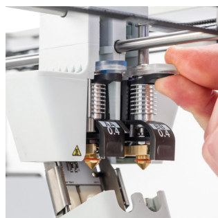
Print core BB 0.4、0.8 毫米 专为打印可溶性支撑材料设计而成
