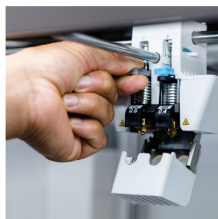
Print core CC 0.6 毫米 红宝石材质，用于打印研磨性复合材料
